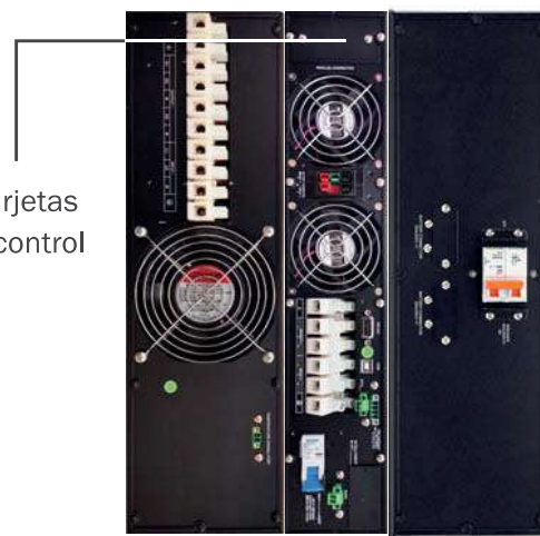
Transformador de aislamiento Módulo de control Banco de baterías
